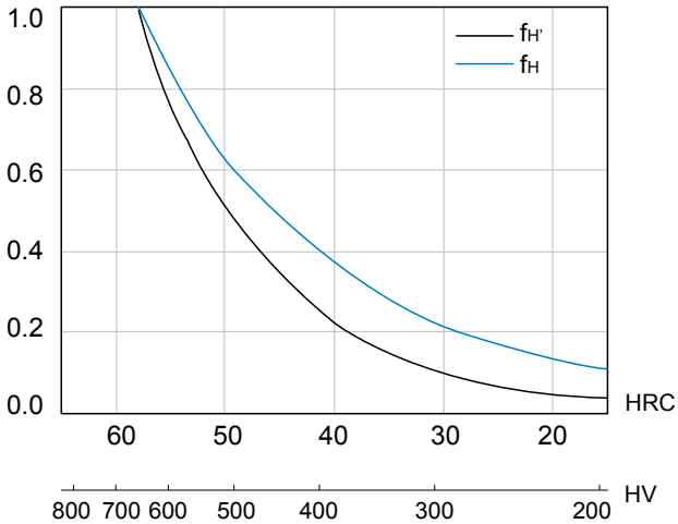
図31. 硬さ係数
