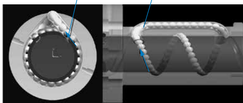
FSVH循環経路（新製品）
