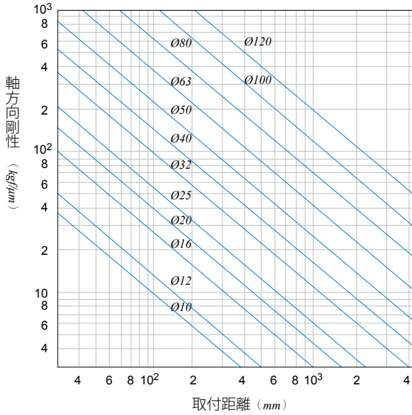
図17. ボールねじ軸の剛性 (固定-自由)
