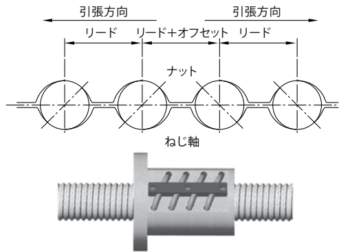
図22. オフセット予圧
