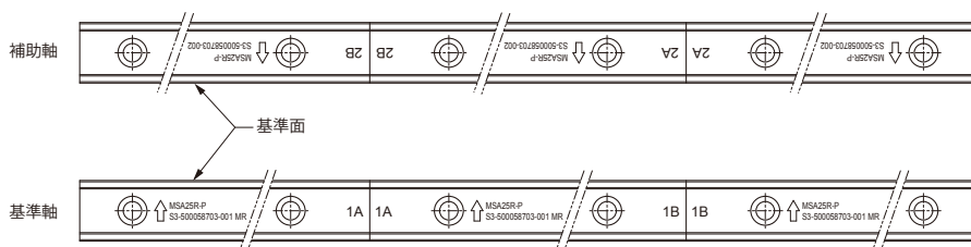
図8. 接続レール
